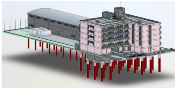
新研修所のB I Mモデル
