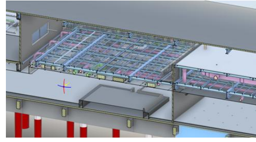
新研修所のB I Mモデル
